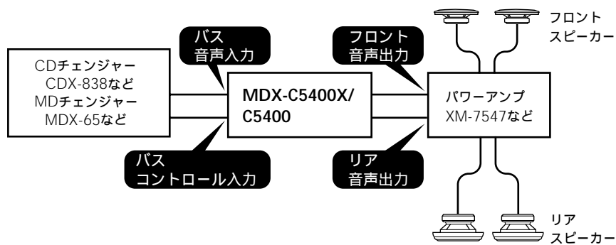
接続例1
