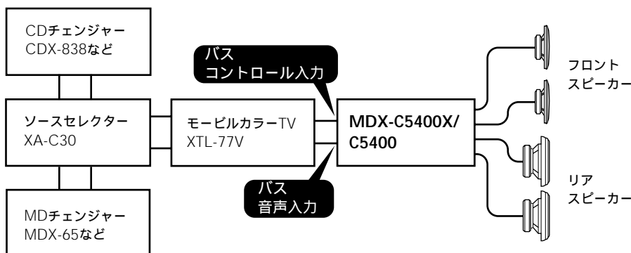
接続例2
